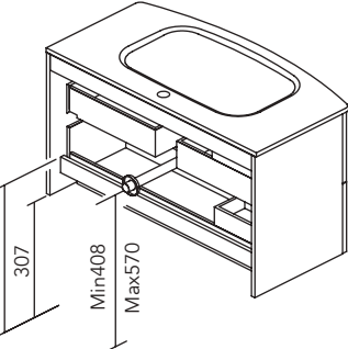
2 cajones. Fondo tubería 7 cm.
