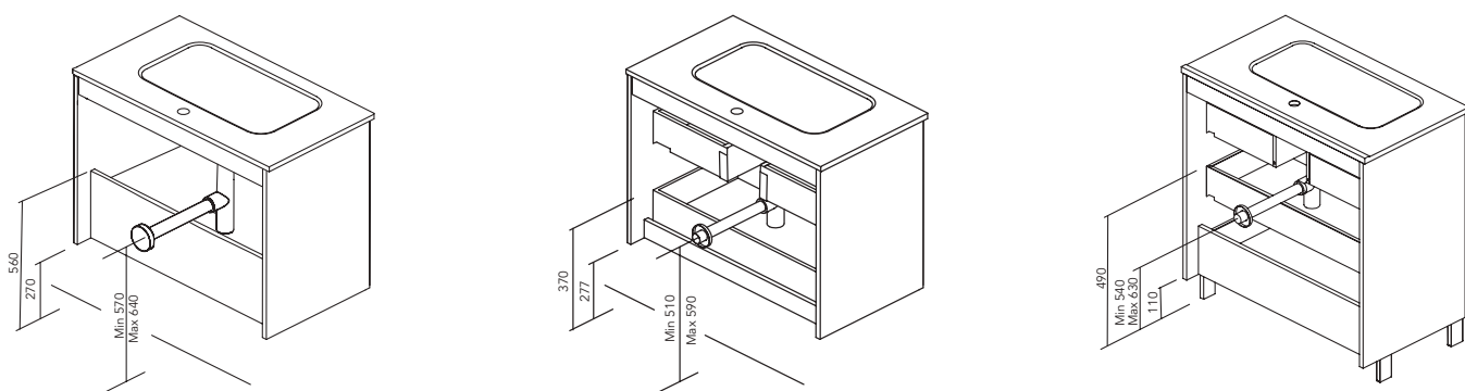
2 puertas. Fondo tubería 7 cm.
