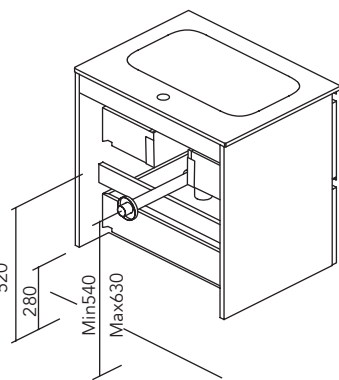
2 cajones. Fondo tubería 7 cm.
