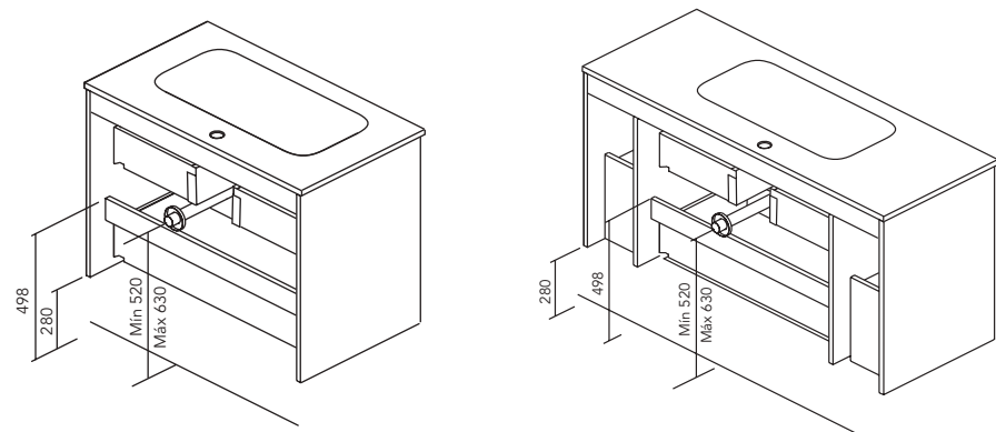
2 cajones. Fondo tubería 7 cm.
