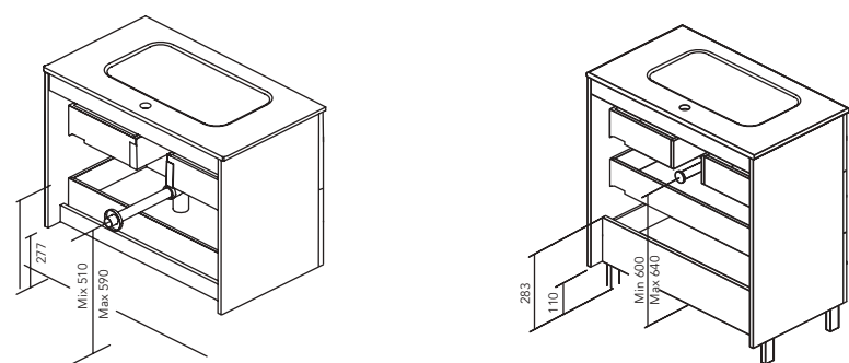
2 cajones. Fondo tubería 7 cm
